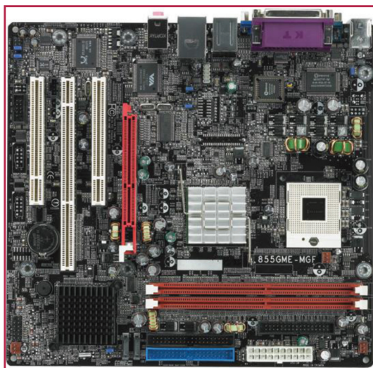
شکل ۱-۷- برد اصلی
